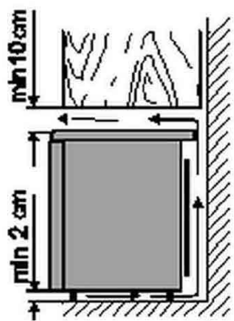
Abb. 2: Ansicht seitlich
