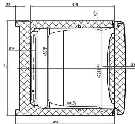
Abb. 3: Ansicht von oben mit geöffneter Gerätetür
