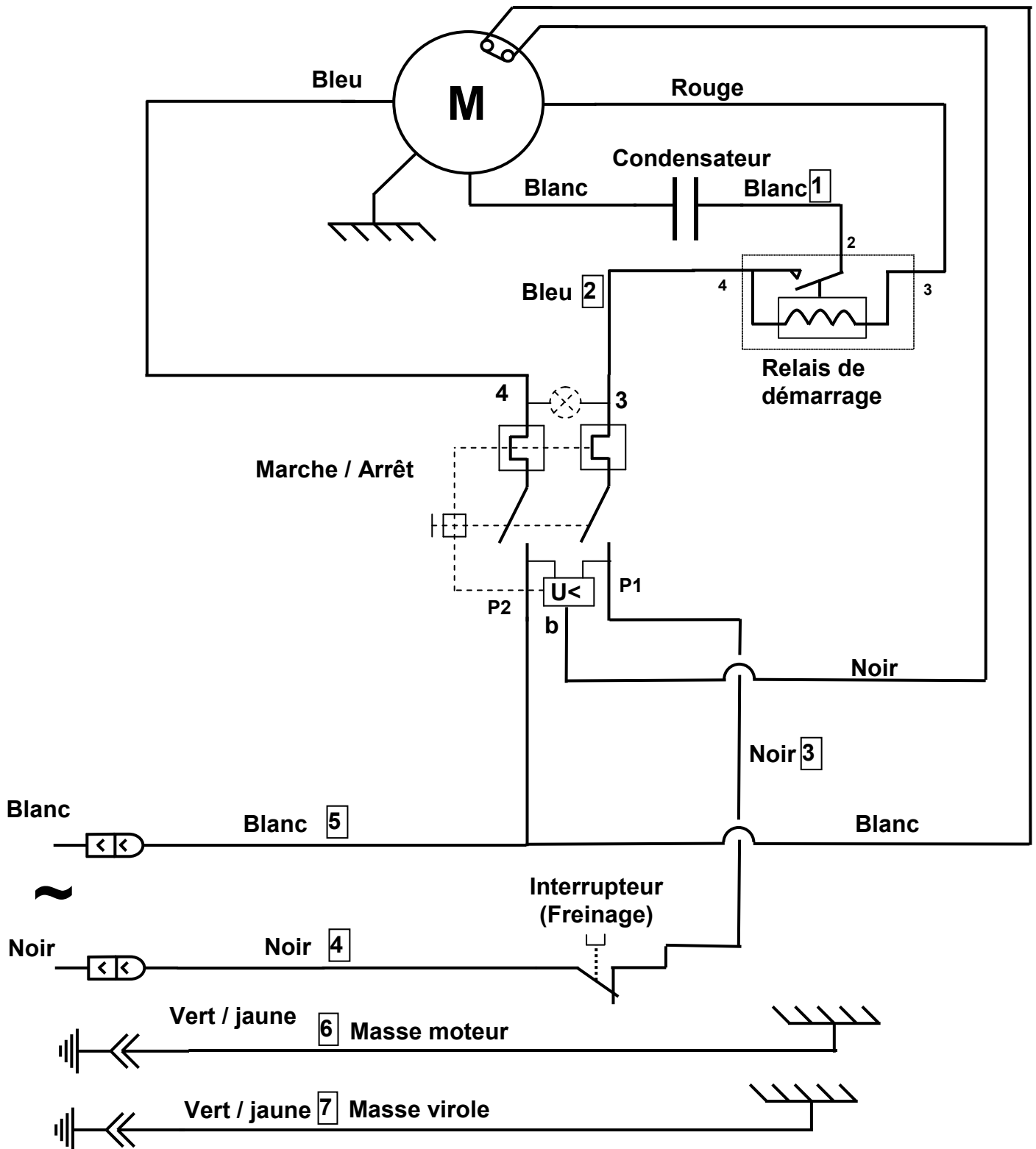
Schéma électrique : 100-120V 50/60Hz
