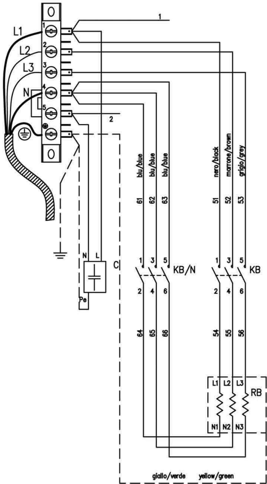
400-415 3P+N 50/60Hz
